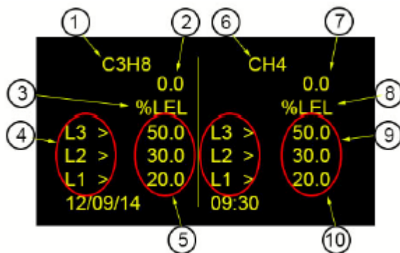
Рисунок 2-5: Двойной дисплей для отображения информации по газу
