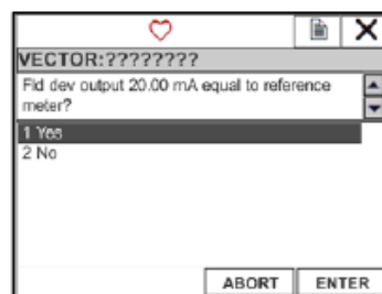
Рисунок 5-39: Подтверждение калибровки тока 20 мА
