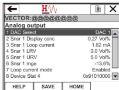
Рисунок A2-5: Меню аналогового выхода
