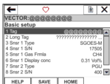
Рисунок A2-8: Меню базовых настроек
