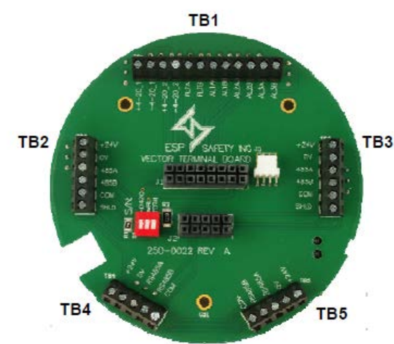
Рисунок 4-9: Клеммная колодка
