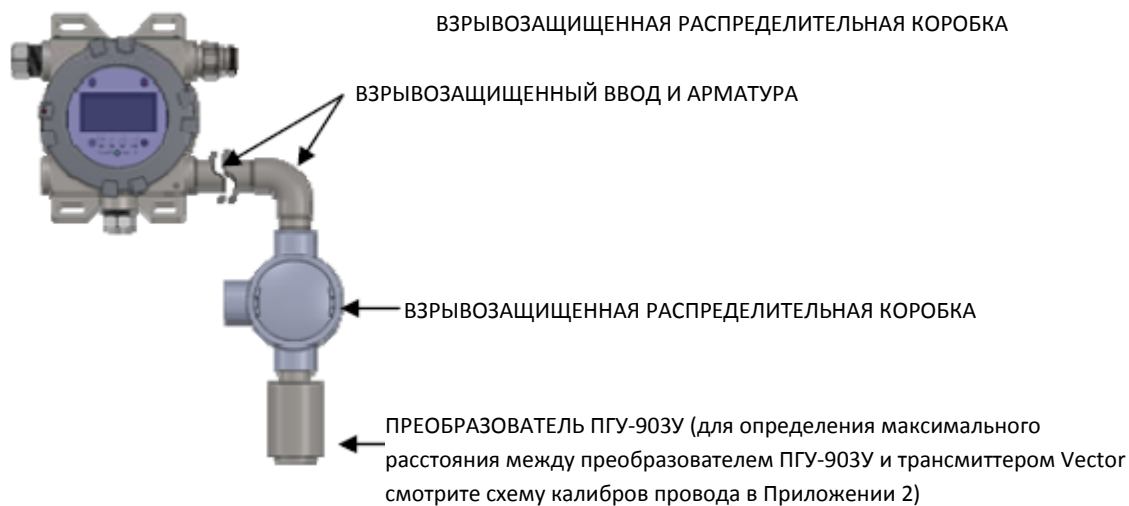
РИСУНОК 4-1: УДАЛЕННАЯ КОНФИГУРАЦИЯ
