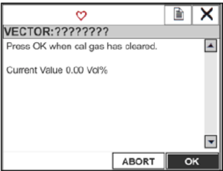
Рисунок 5-17: Выход из режима нулевой калибровки
