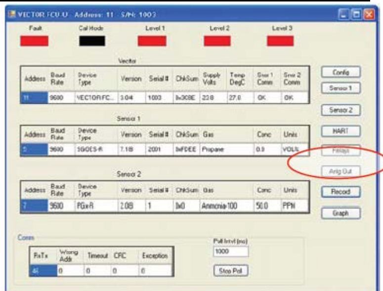
Рисунок 5-28: Основная форма Vector
