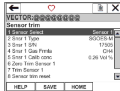
Рисунок A2-6: Меню подстройки преобразователя ПГУ-903У:
