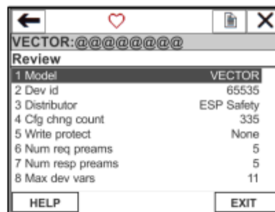
Рисунок A2-19: Меню просмотра
