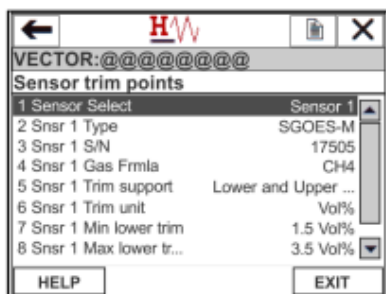
Рисунок A2-4: Меню точек подстройки преобразователя ПГУ-903Уа
