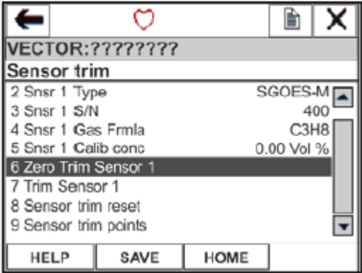
Рисунок 5-12: Экран подстройки преобразователя ПГУ-903У (Ноль)
