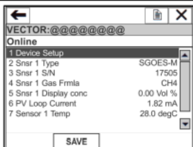
Рисунок A2-1: Меню Online
