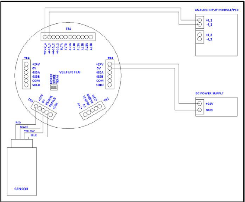
Рисунок 4-10: Проводка Vector для модуля аналогового ввода с токовыми входами и одним преобразователем ПГУ-903У
