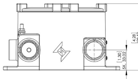
Рисунок 1-3: Габаритные размеры блока управления Vector
