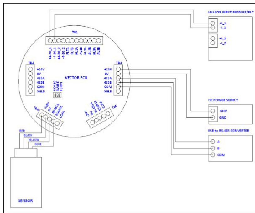
Рисунок 4-15: Подключение Vector к RS-485, программе управления ESP или SCADA
