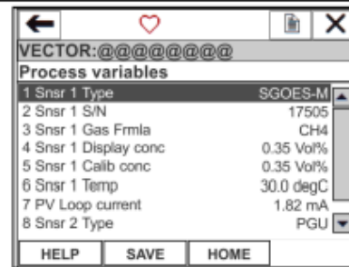
Рисунок A2-3: Меню параметров процесса
