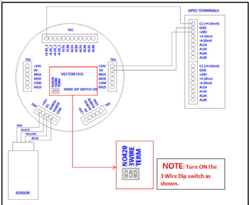
Рисунок 4-11: Подключение газоанализатора Vector ко вторичному устройству S
